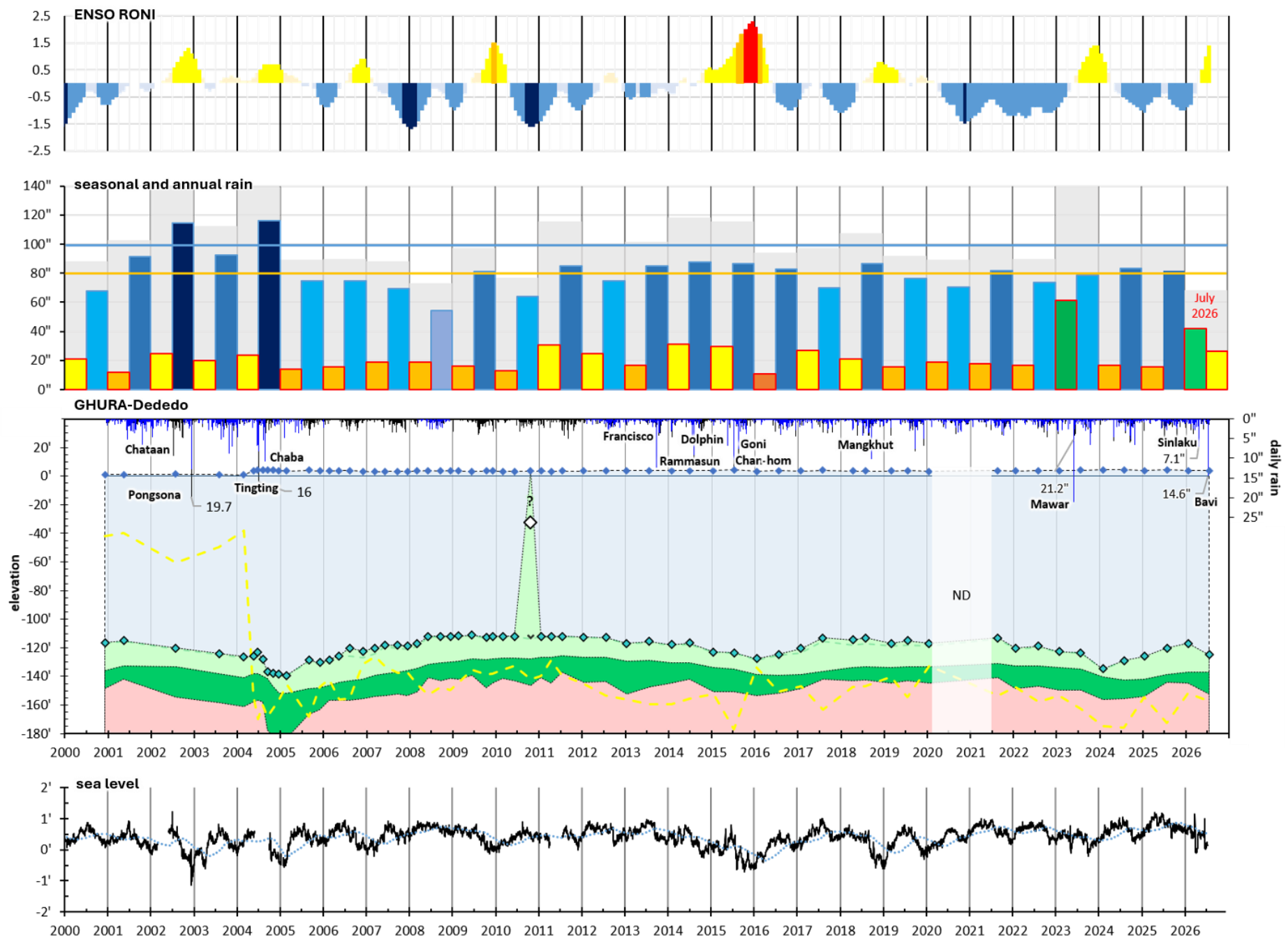
GHURA-Dededo DOW phreatic hydrograph (WERI TR 189)
